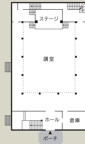
平面図 (1階：367㎡)
